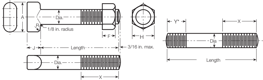
Stud Bolt
